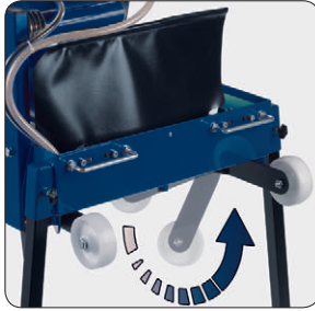
Inklapbare transportwielen
