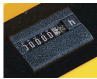
Urenteller standaard. Voor de DF serie is de garantie 8760 draaiuren, maximaal 3 jaar.
