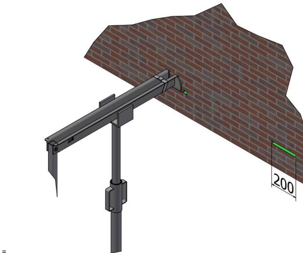
Figuur 6: Weergave van muursleuven.
